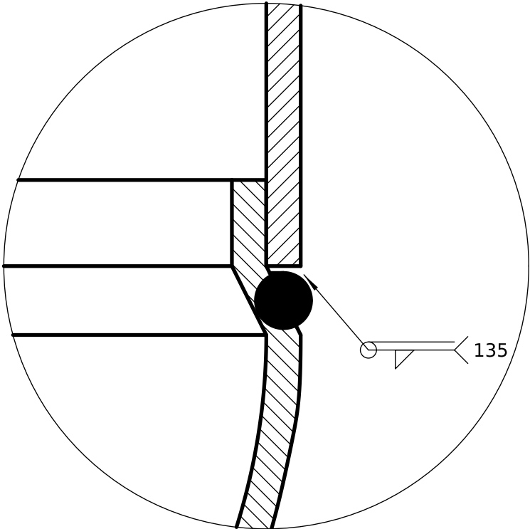
DETALLE D (2:1) Casquete inferior con borde reducido
