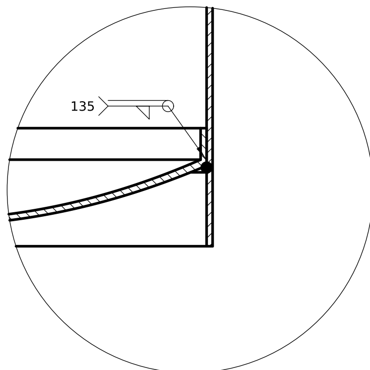
DETALLE D (1:1) Fondo encastrado y pollera
