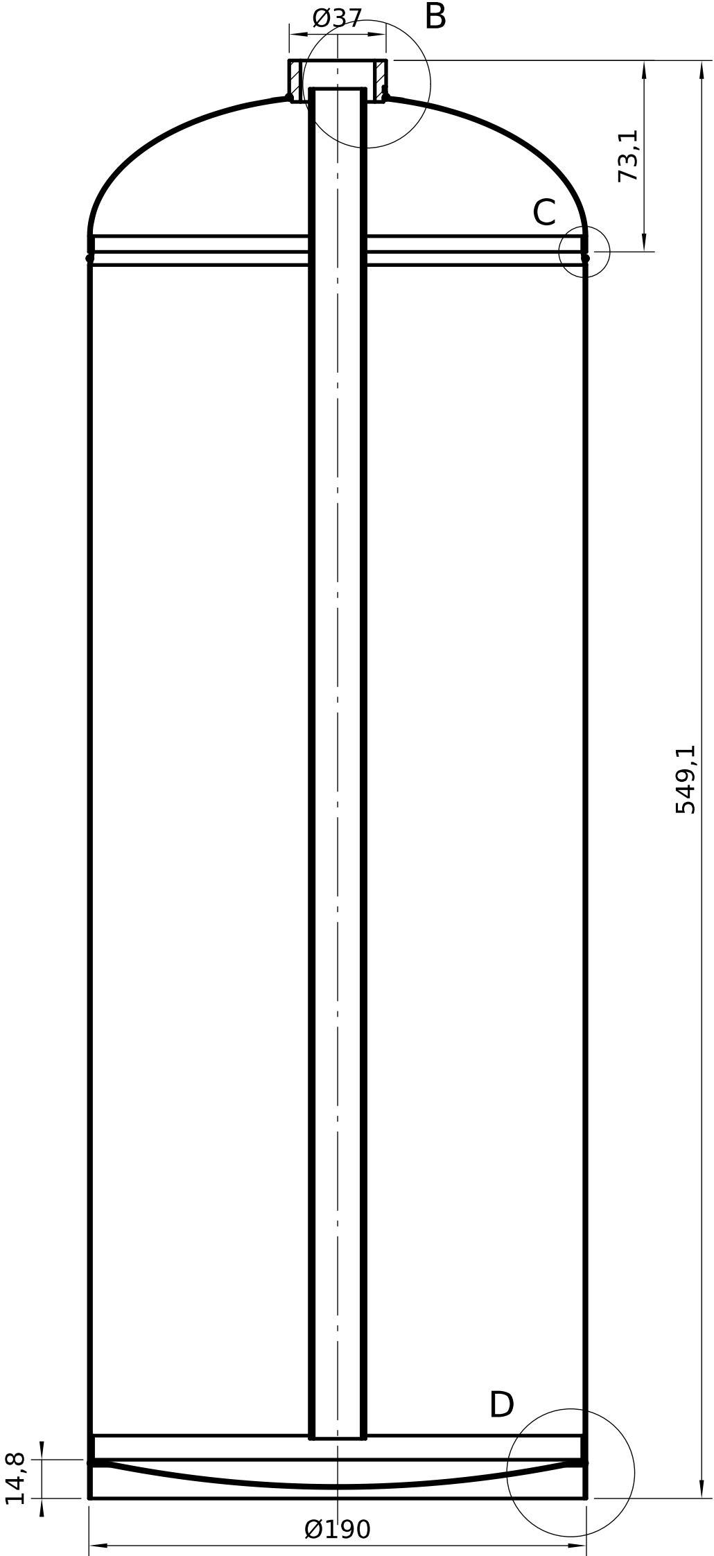
CORTE A-A (1:2)
