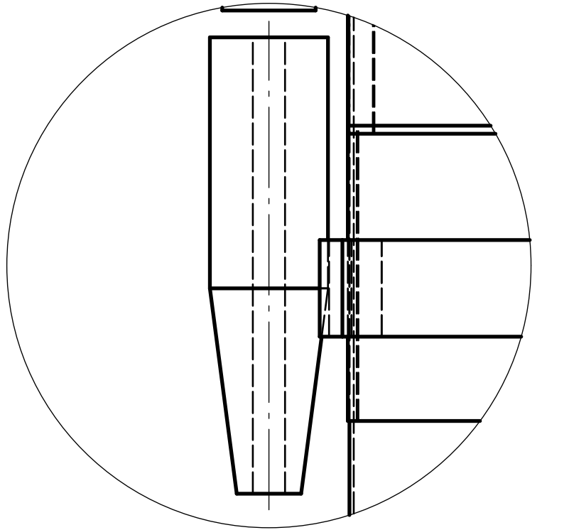
DETALLE E (1:1) Tobera de chorro pleno
