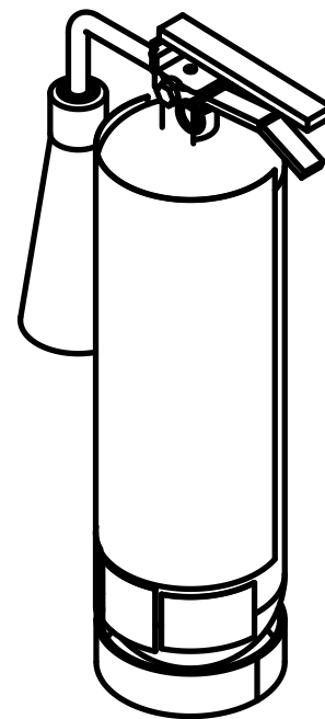
ISOMETRÍA (ESC. 1:5)
