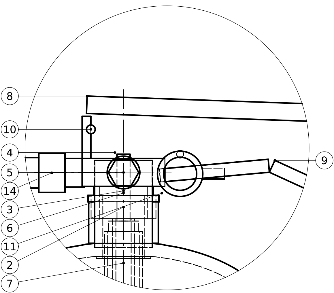
DETALLE A (1:1) Válvula, disco de seguridad y manijas
