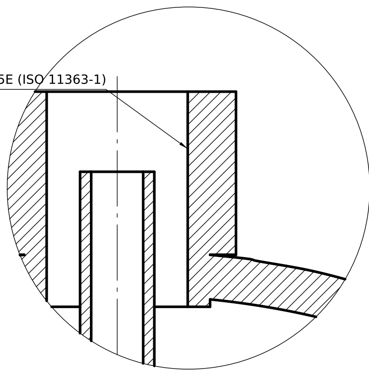
DETALLE B (2:1) Cuello roscado
