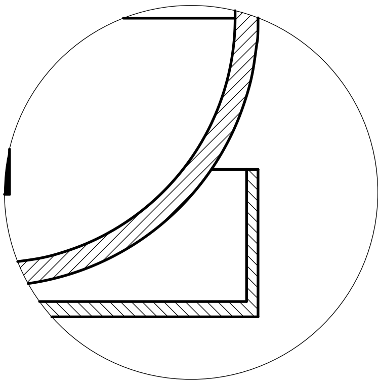
DETALLE D (1:1) Fondo y pie de apoyo
