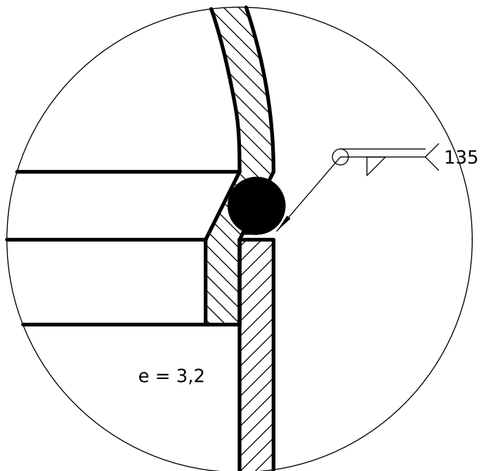
DETALLE C (2:1) Casquete con borde reducido y tope labio 8 dentro del cuerpo, escalón 6,4 x e 3,2; cordón en el escalón
