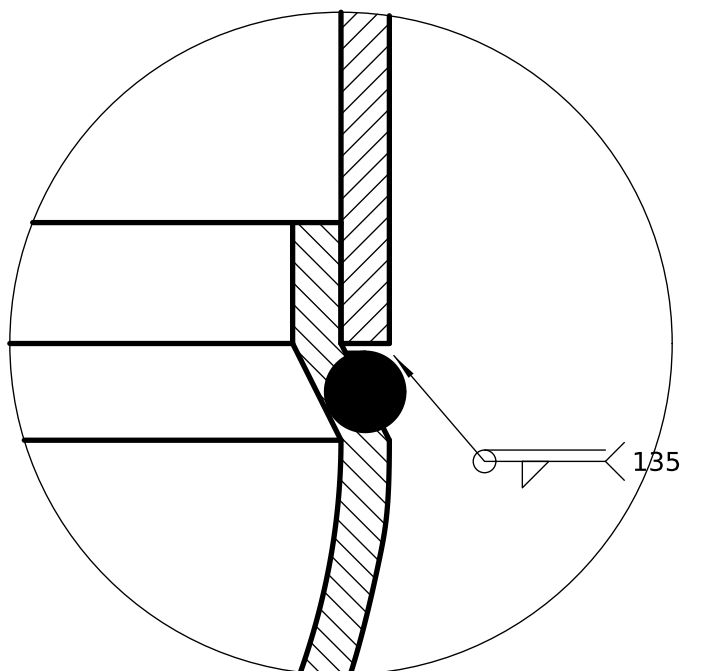
DETALLE D (2:1) Casquete inferior con borde reducido labio 8, escalón 6,4; mismo casquete que la cúpula
