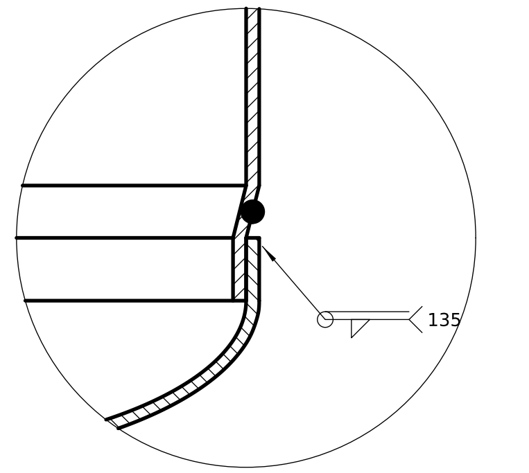
DETALLE D (2:1) Bordón inferior y fondo caño con los dos extremos reducidos: escalón e 1,25 x 5, labio 6
