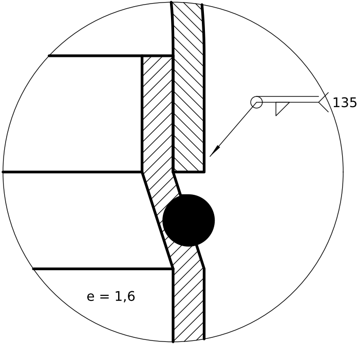
DETALLE C (5:1) Bordón del cuerpo y cúpula escalón e 1,6 x 5, labio 6 (bordoneadora); cúpula por fuera
