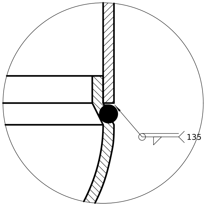
DETALLE D (1:1) Casquete inferior con borde reducido labio 11,9, escalón 9,5; mismo casquete que la cúpula
