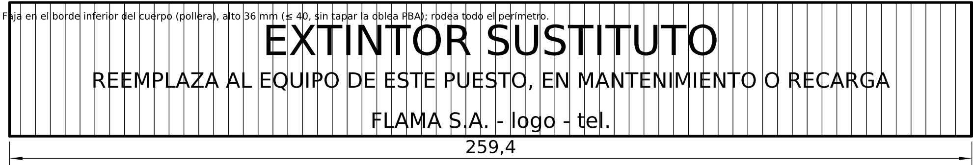
DETALLE 1 - DESARROLLO DE LA FAJA 36 × 259 (esc. 1:1) - amarillo; leyendas negras repetidas
