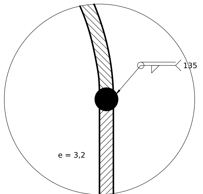
DETALLE C (2:1) Unión cúpula-cuerpo
