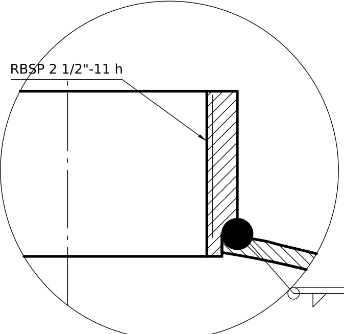
DETALLE B (1:1) Cuello roscado
