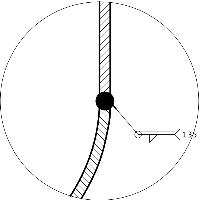
DETALLE D (1:1) Unión fondo-cuerpo
