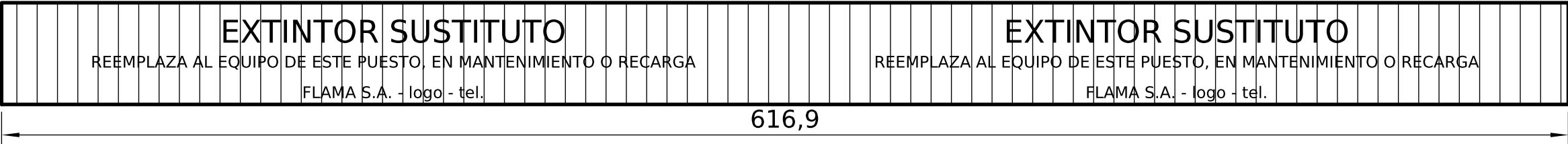
DETALLE 1 - DESARROLLO DE LA FAJA 40 × 617 (esc. 1:2) - amarillo; leyendas negras repetidas
