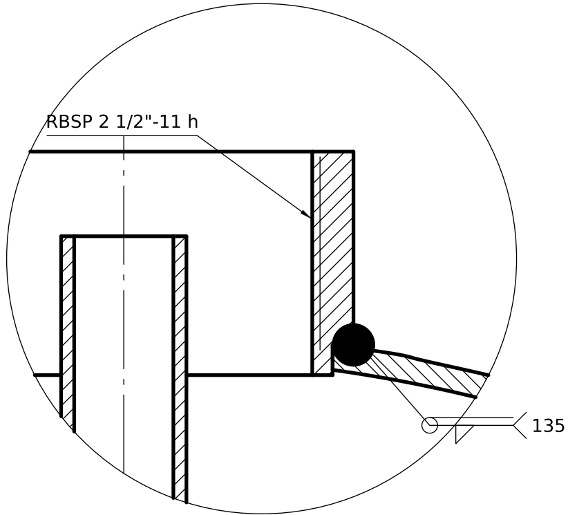
DETALLE B (1:1) Cuello roscado
