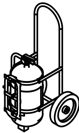
ISOMETRÍA (ESC. 1:20)
