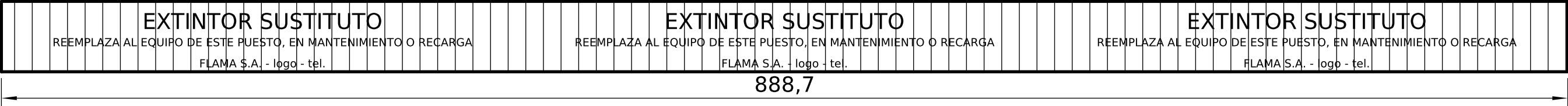
DETALLE 1 - DESARROLLO DE LA FAJA 40 × 889 (esc. 1:2.5) - amarillo; leyendas negras repetidas
