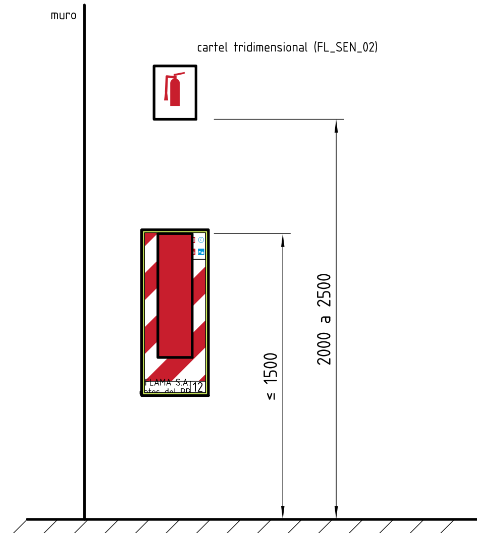
PUESTO DE INCENDIO (1:20)
