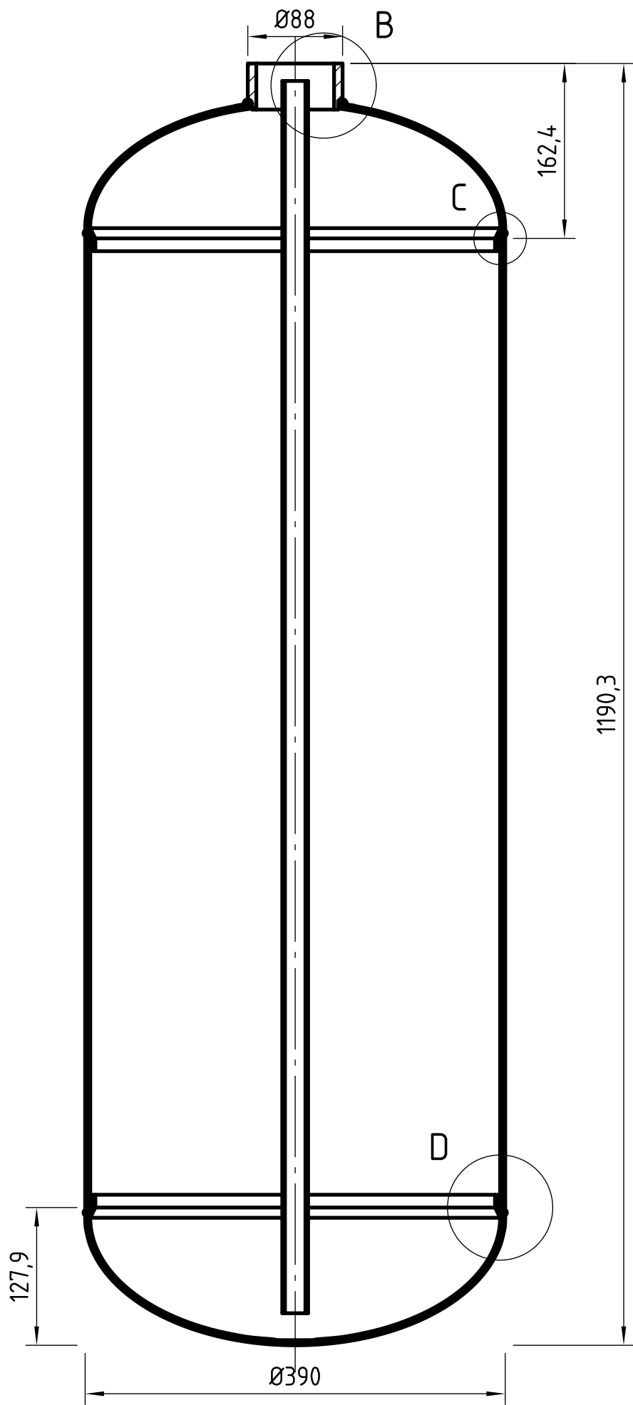
CORTE A-A (1:5)
