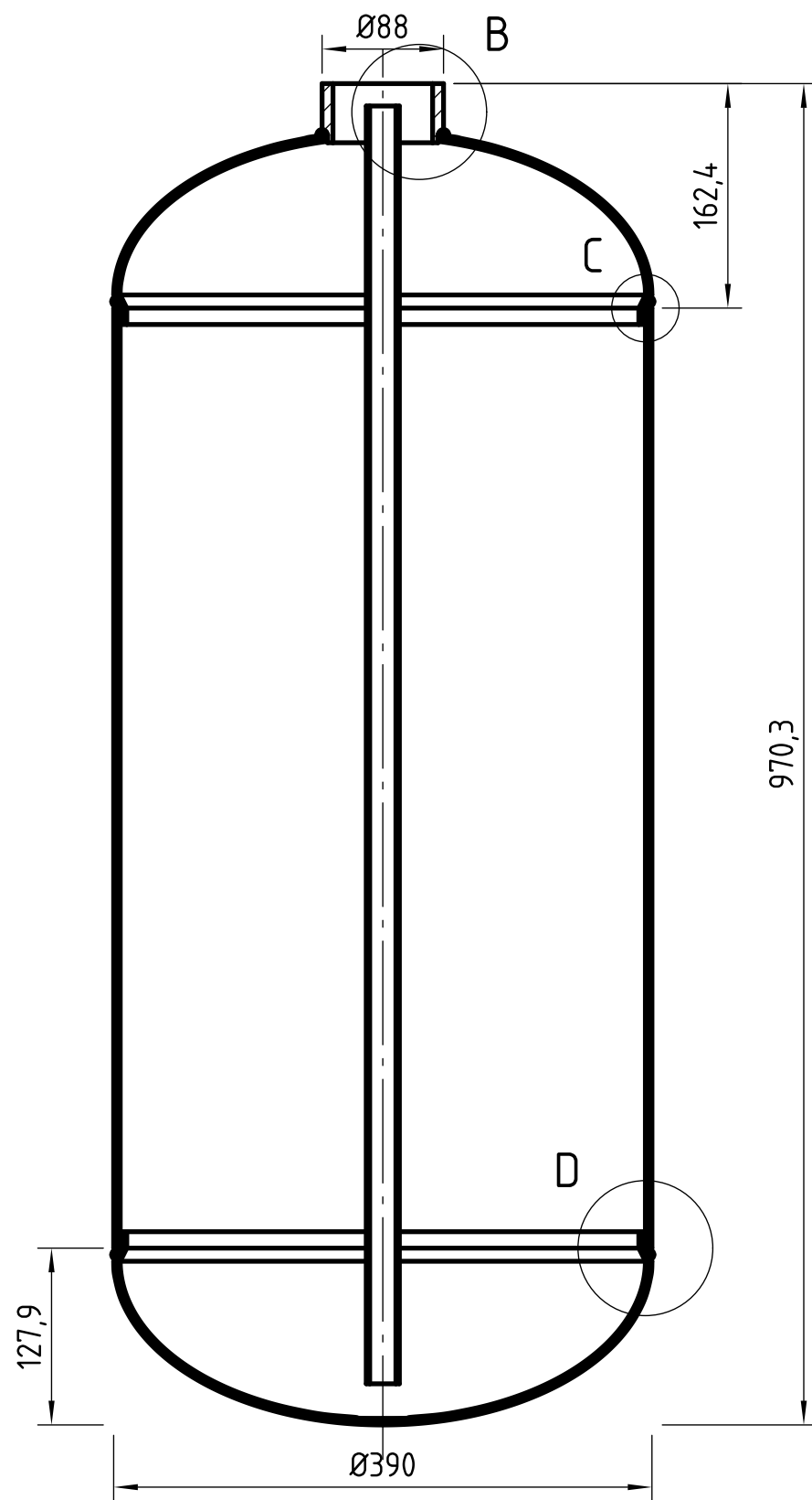
CORTE A-A (1:5)
