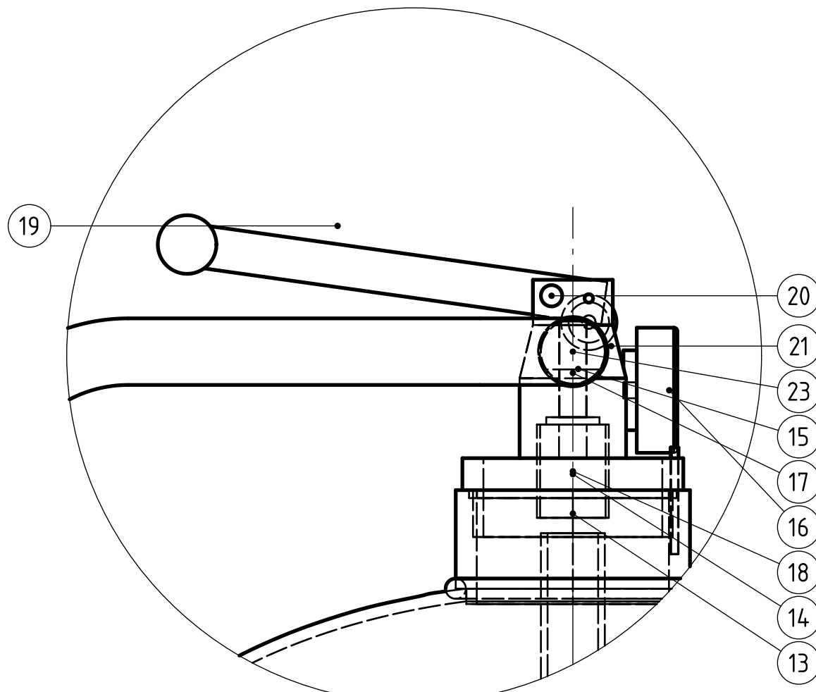
DETALLE A (1:2) Válvula, manómetro y palanca (vista lateral)
