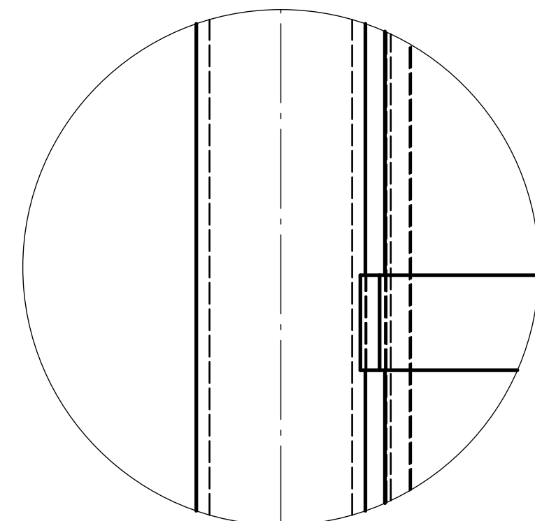
DETALLE E (1:1) Lanza espumígena
