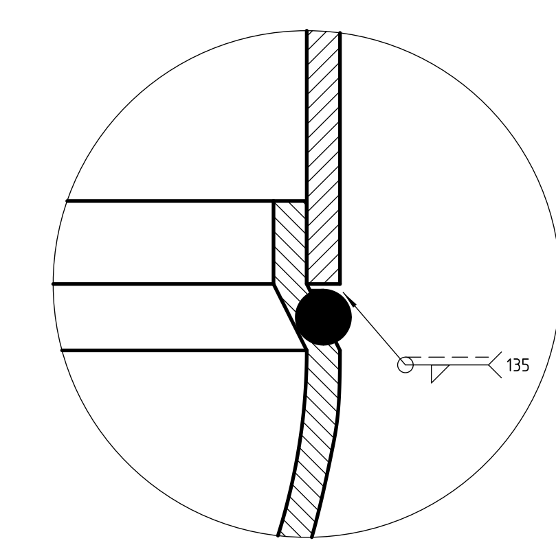
DETALLE D (2:1) Casquete inferior con borde reducido
