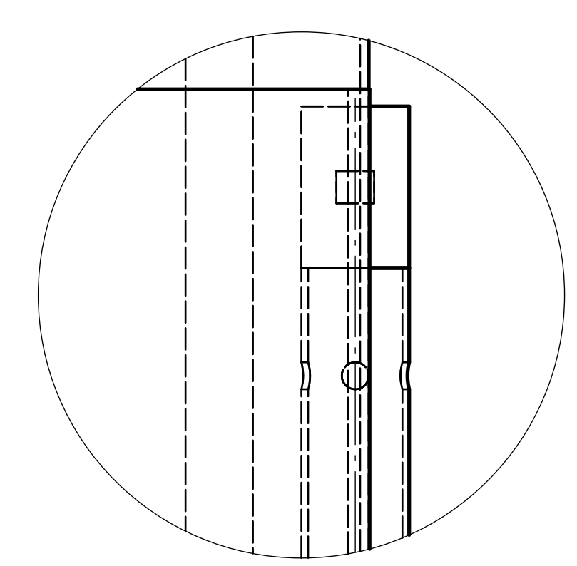
DETALLE E (1:2) Válvula esférica y tobera
