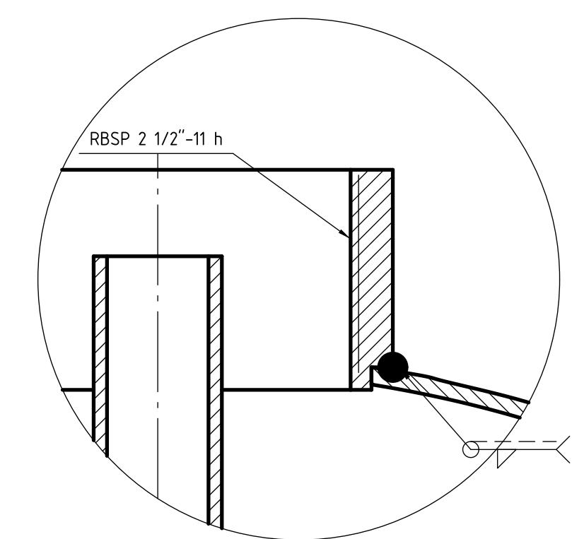
DETALLE B (1:1) Cupla soldada
