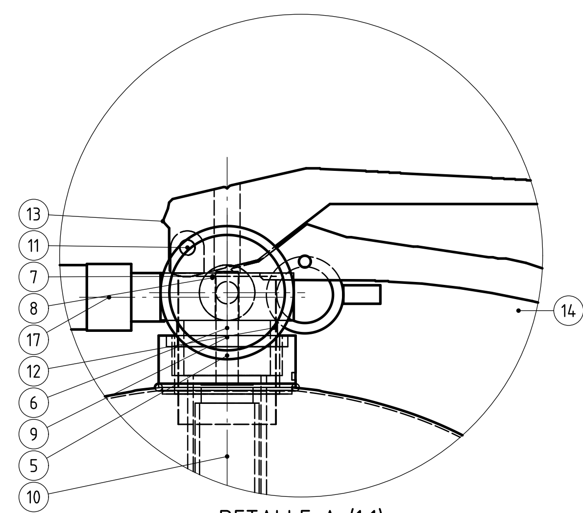
DETALLE A (1:1) Válvula, manómetro y manijas
