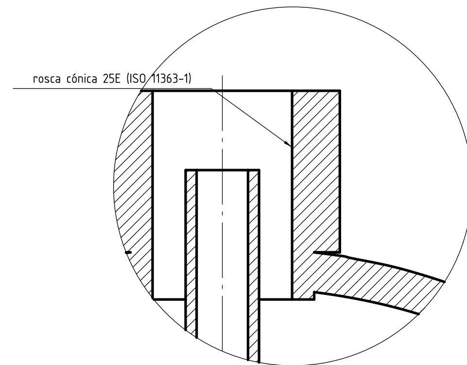
DETALLE B (2:1) Cuello roscado
