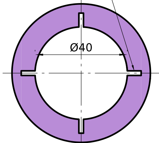
PLANTA - anillo plano (1:1) color 2026 (dígito 6): LILA
