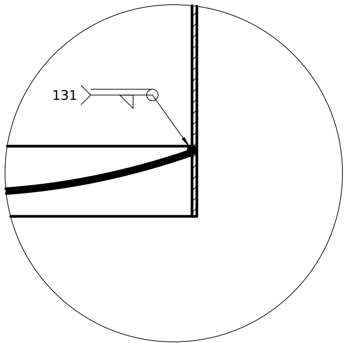
DETALLE D (1:1) Fondo y pollera
