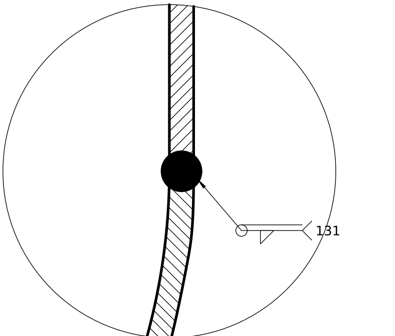
DETALLE D (2:1) Unión fondo-cuerpo
