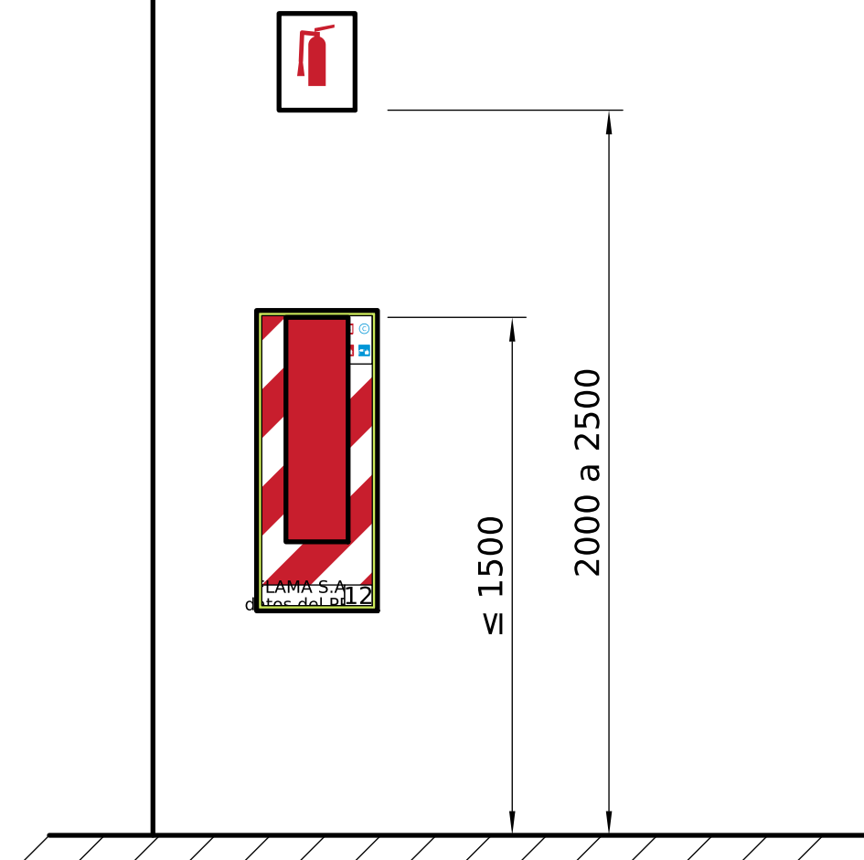
PUESTO DE INCENDIO (1:20)
