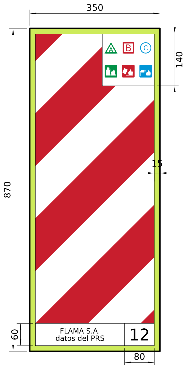
CHAPA 350 × 870 (preferente)
