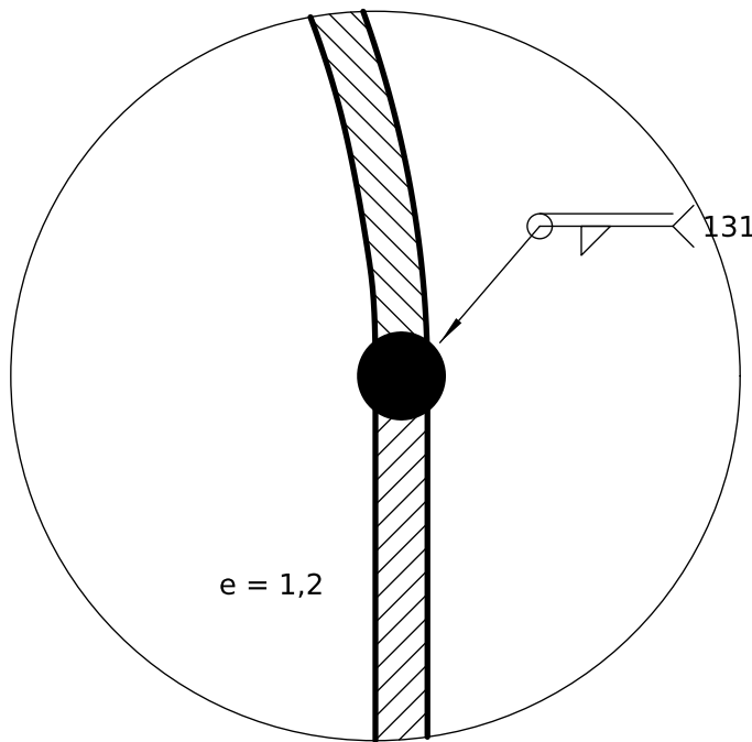
DETALLE C (5:1) Unión cúpula-cuerpo
