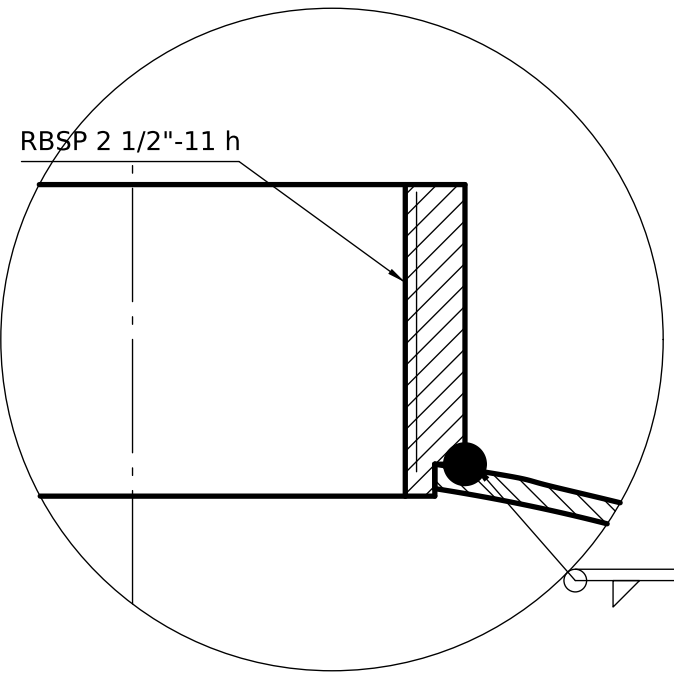
DETALLE B (1:1) Cuello roscado
