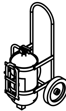
ISOMETRÍA (ESC. 1:20)
