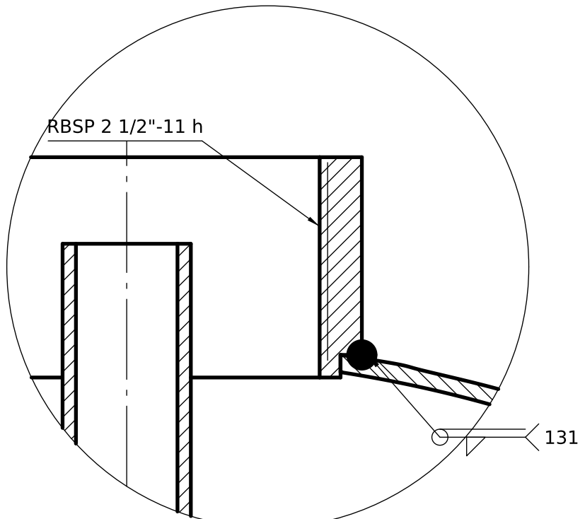
DETALLE B (1:1) Cuello roscado
