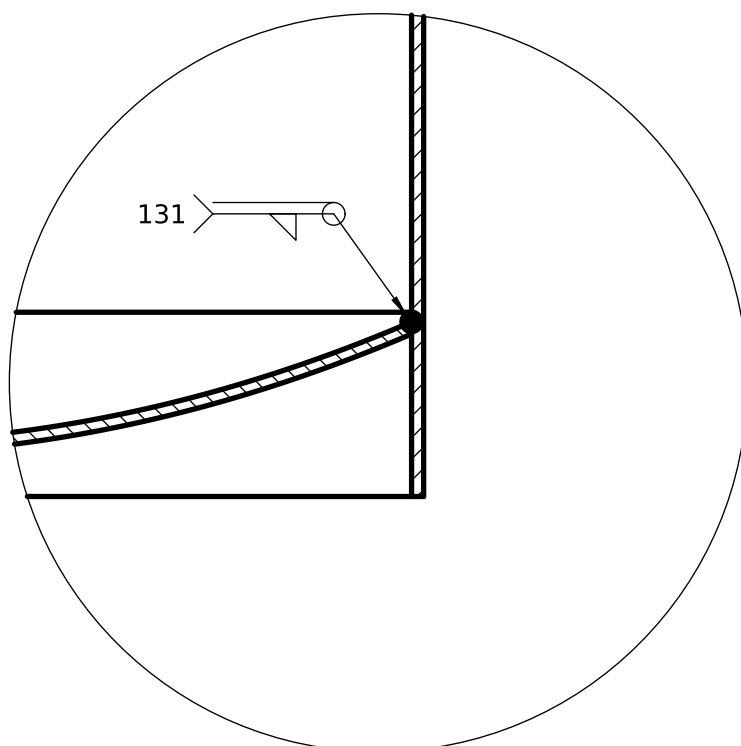
DETALLE D (1:1) Fondo y pollera
