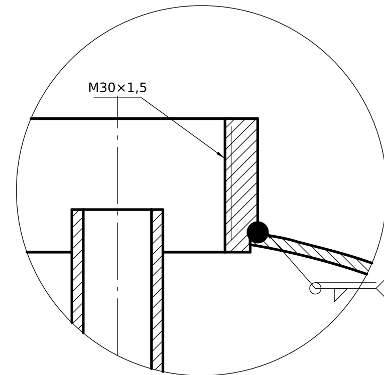
DETALLE B (2:1) Cuello roscado
