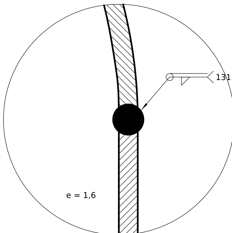
DETALLE C (5:1) Unión cúpula-cuerpo
