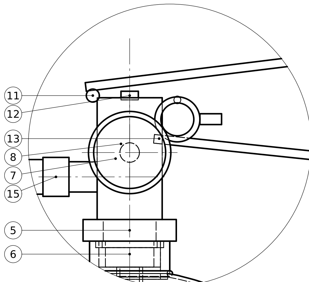
DETALLE A (1:1) Válvula, manómetro y manijas
