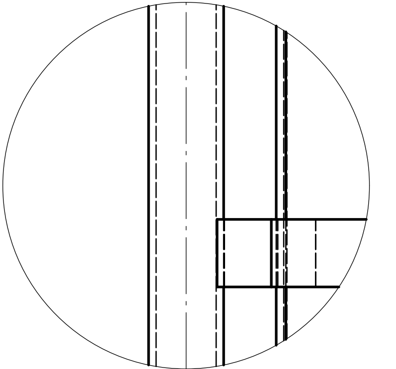
DETALLE E (1:1) Lanza de flujo suave
