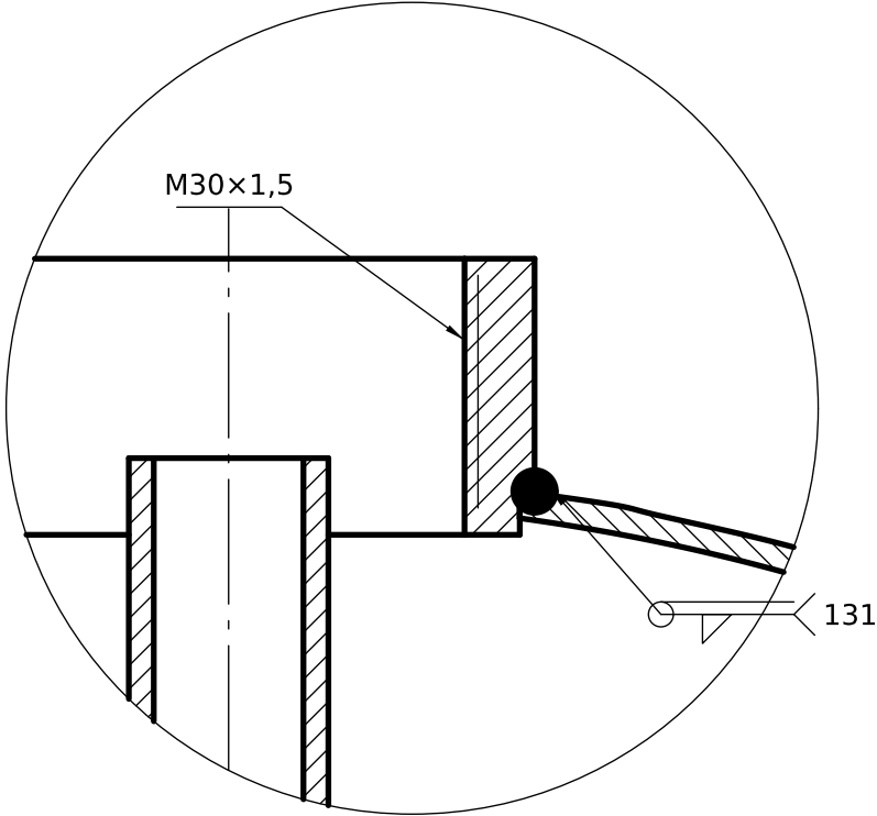
DETALLE B (2:1) Cuello roscado
