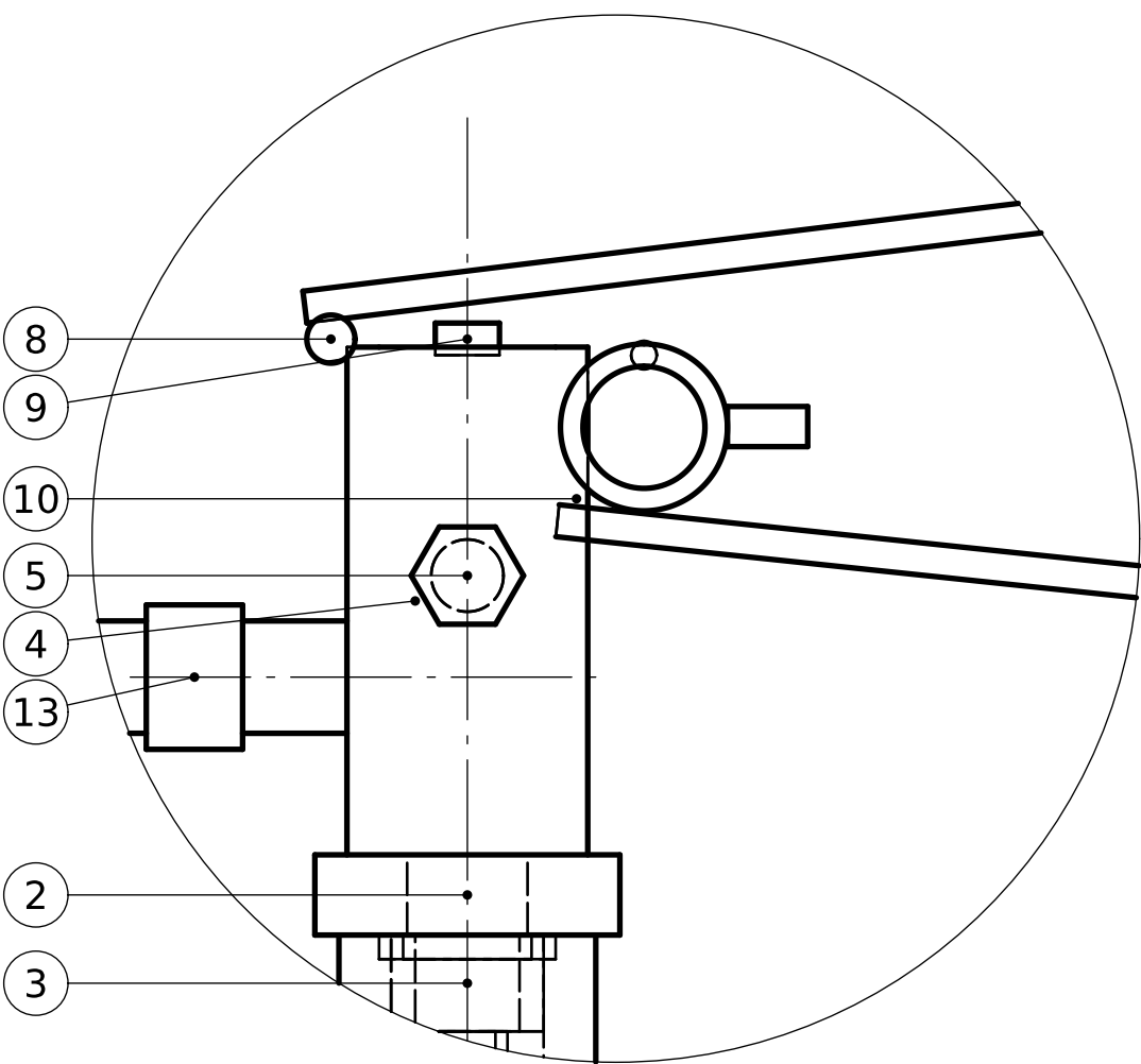
DETALLE A (1:1) Válvula, disco de seguridad y manijas
