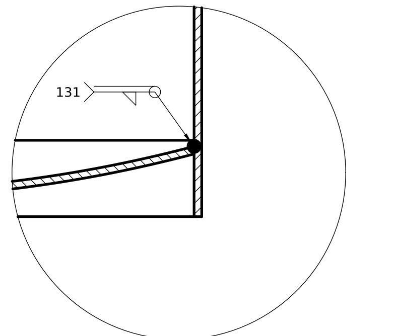
DETALLE D (1:1) Fondo y pollera
