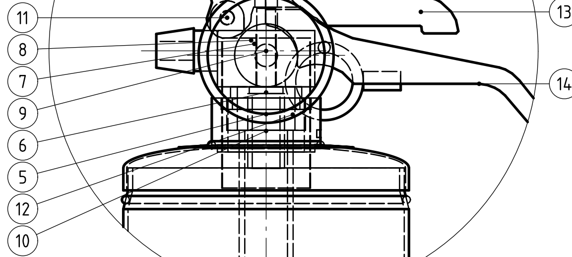
DETALLE A (1:1) Válvula, manómetro y manijas
