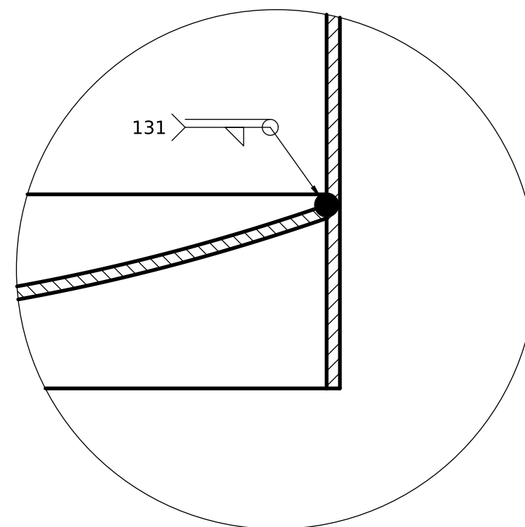
DETALLE D (2:1) Fondo y pollera
