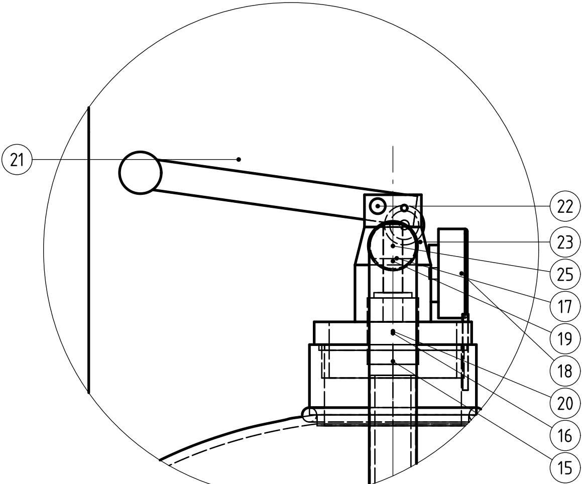
DETALLE A (1:2) Válvula, manómetro y palanca (vista lateral)
