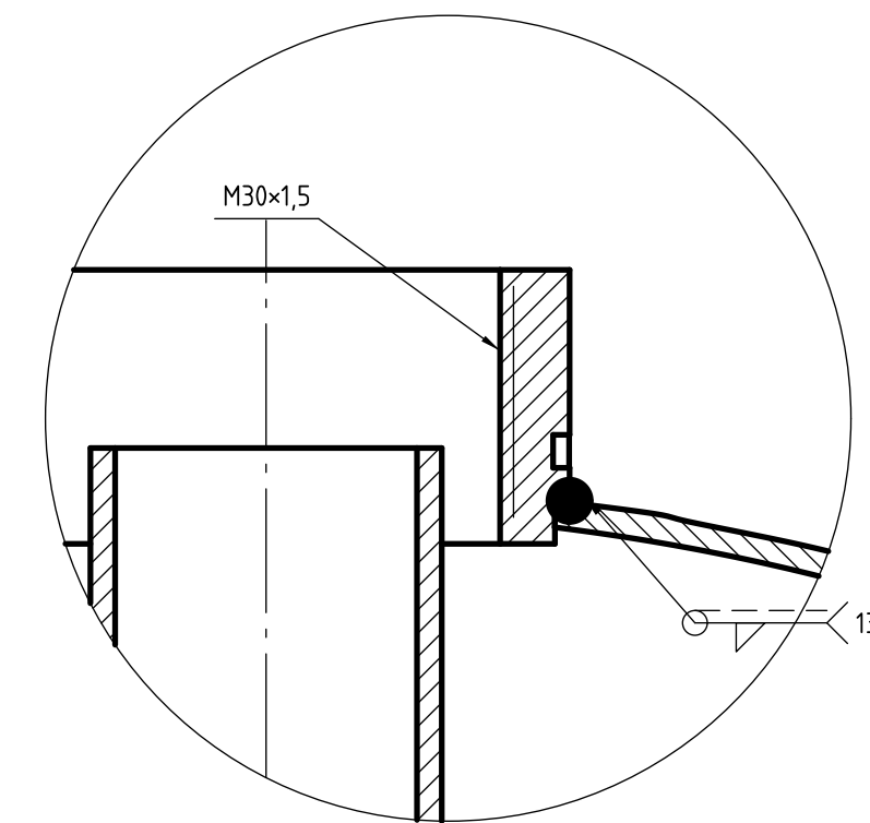
DETALLE B (2:1) Cuello roscado con muesca
