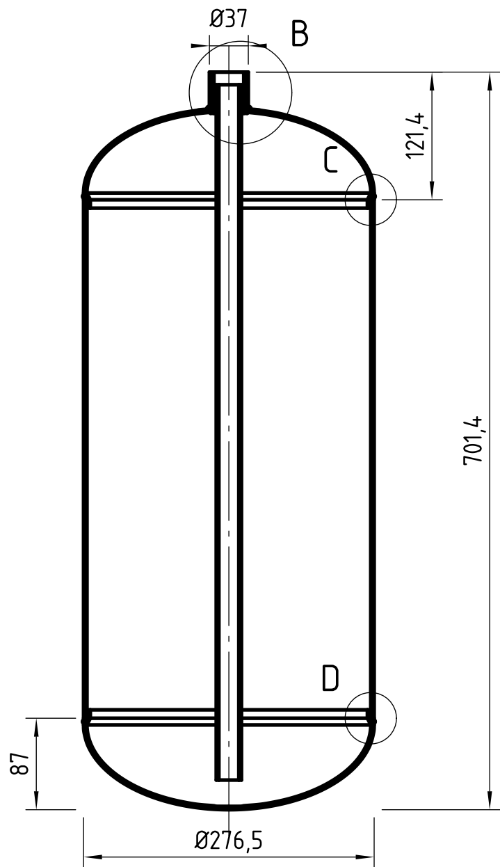
CORTE A-A (1:5)
