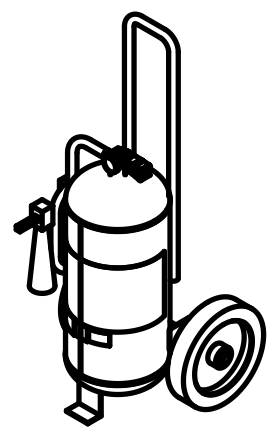
ISOMETRÍA (ESC. 1:20)
