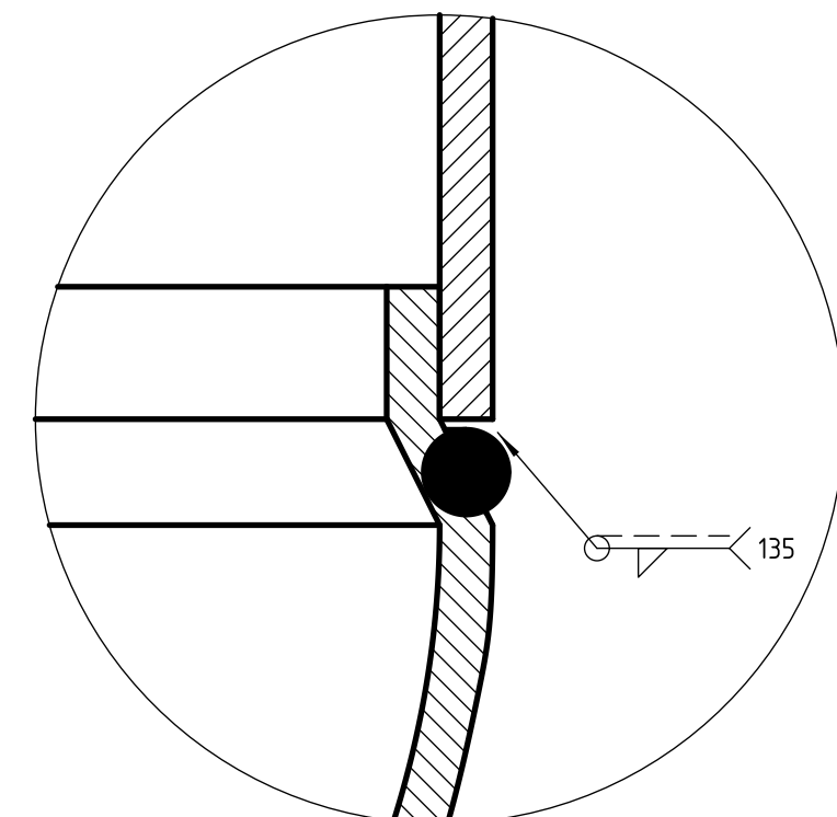
DETALLE D (2:1) Casquete inferior con borde reducido
