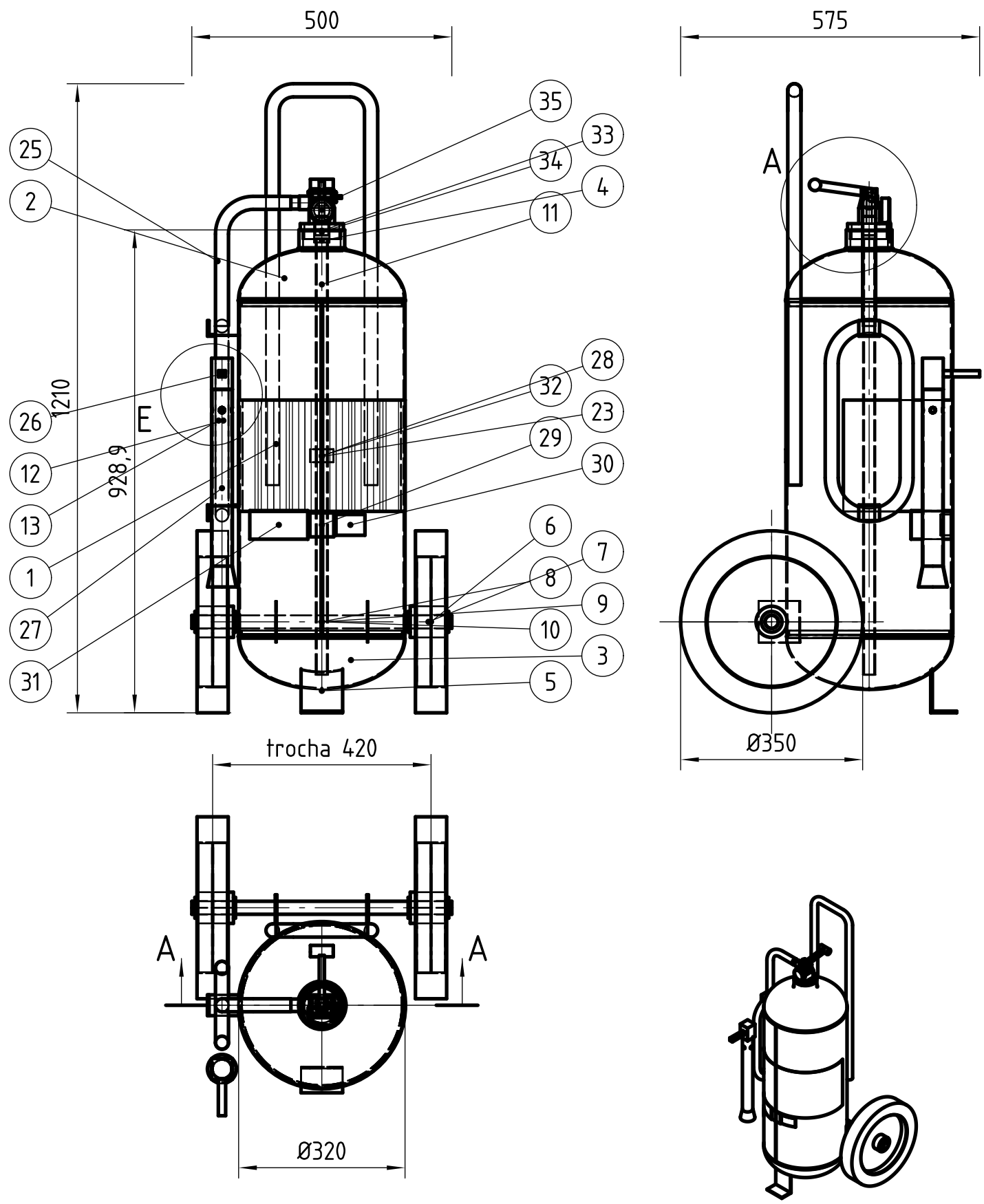
ISOMETRÍA (ESC. 1:20)
