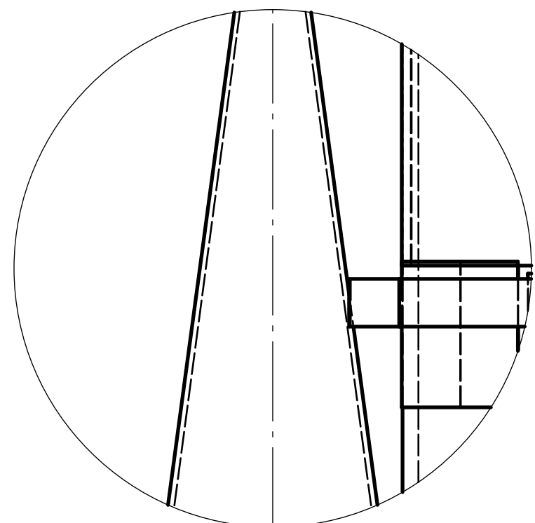
DETALLE E (1:2) Difusor y soporte
