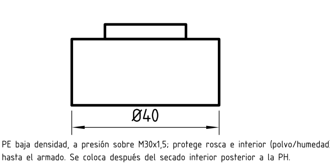
R4 TAPÓN PROTECTOR DE ROSCA
