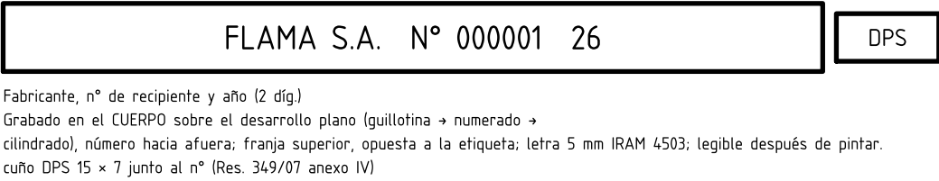
R3 MARCADO GRABADO (IRAM 3523 5.1)
