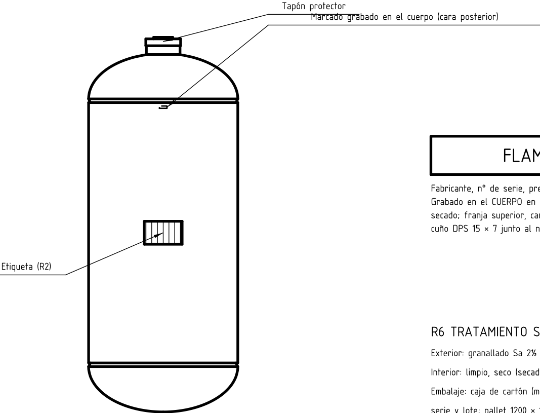
R3 MARCADO GRABADO (IRAM 3550 5.1)
