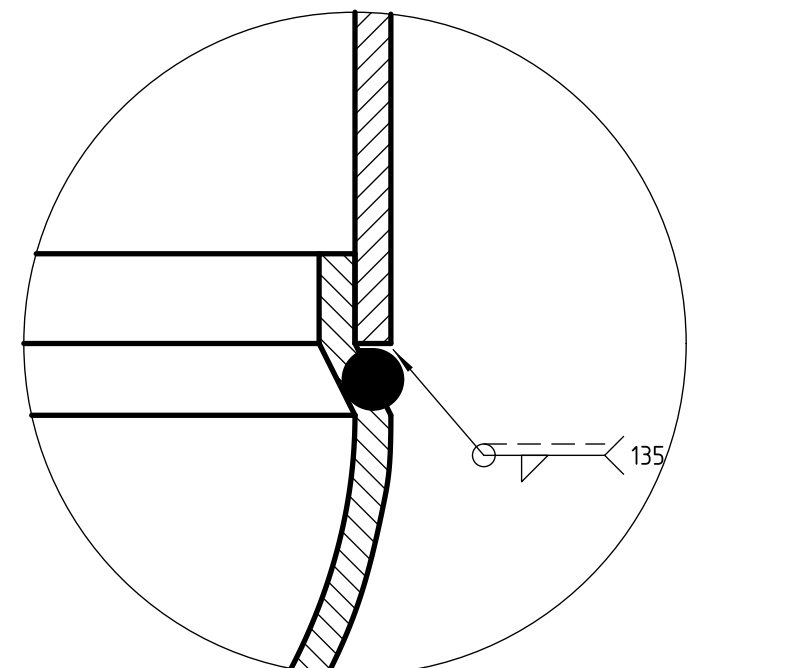
DETALLE D (1:1) Casquete inferior con borde reducido labio 11,9, escalón 9,5; mismo casquete que la cúpula
