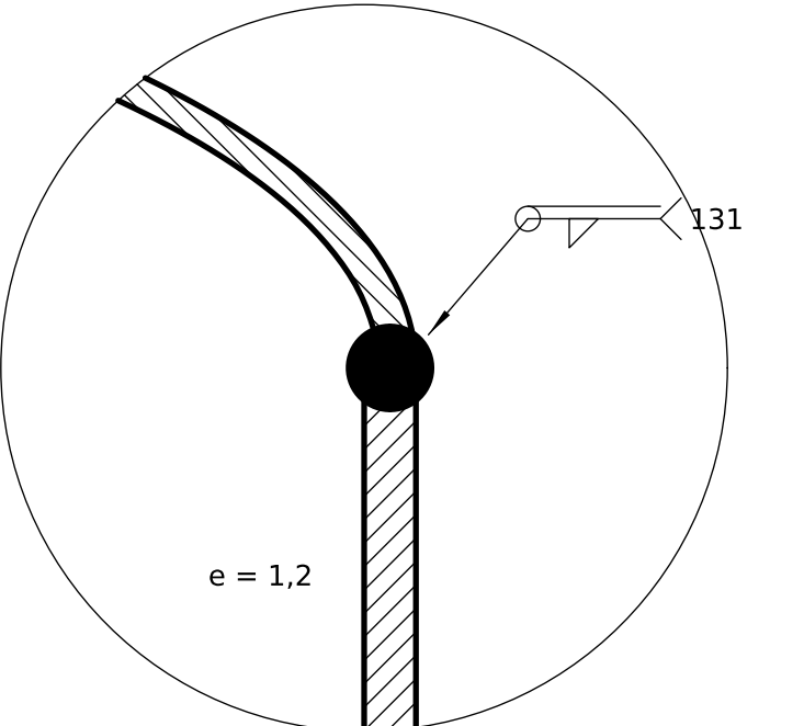
DETALLE C (5:1) Unión cúpula-cuerpo
