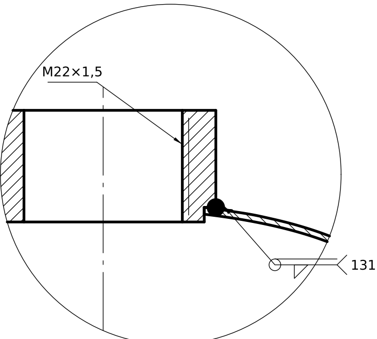
DETALLE B (2:1) Cuello roscado
