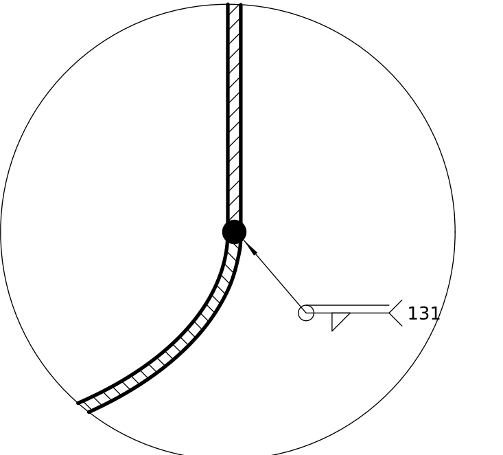
DETALLE D (2:1) Unión fondo-cuerpo
