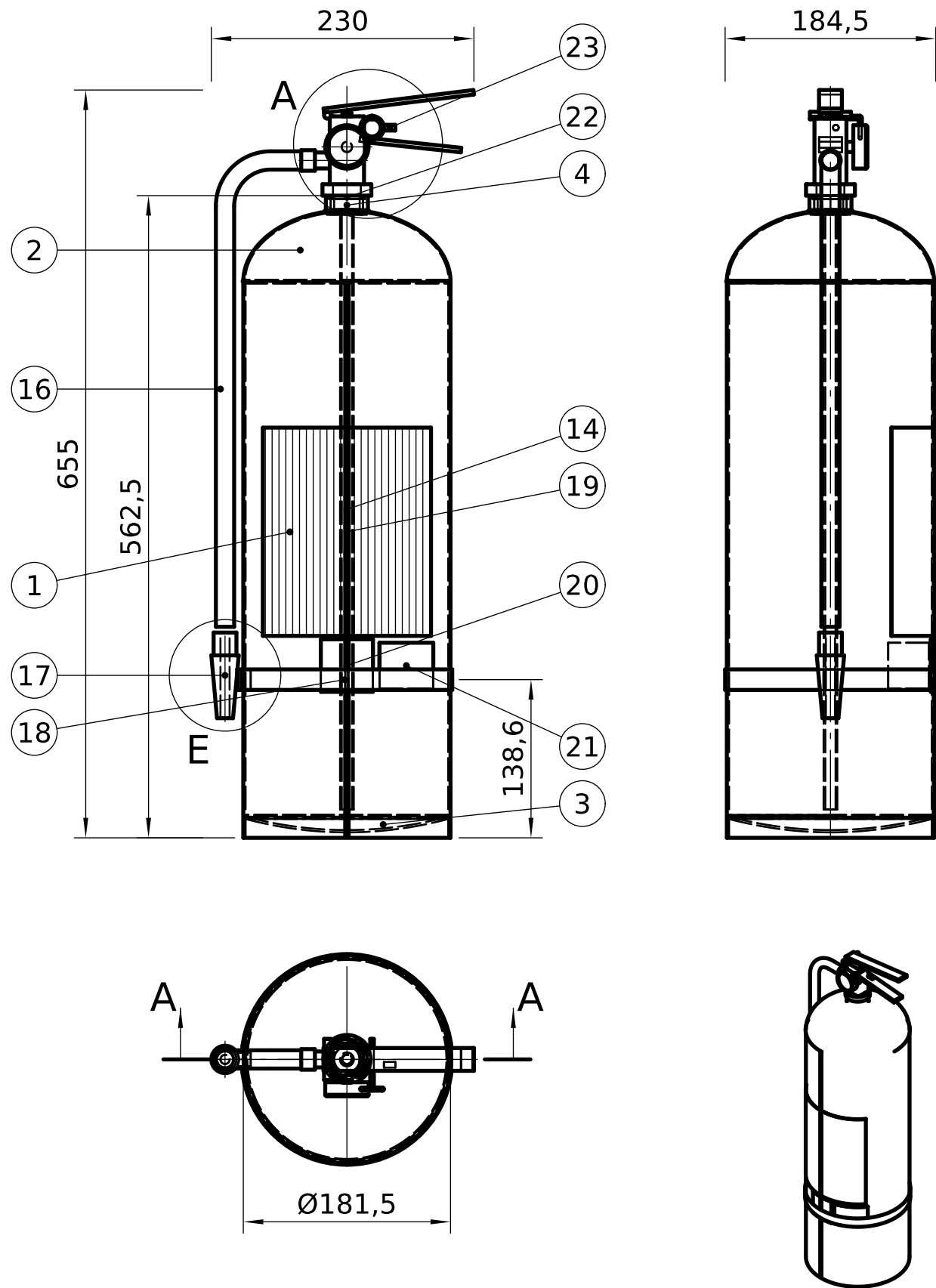
ISOMETRÍA (ESC. 1:10)
