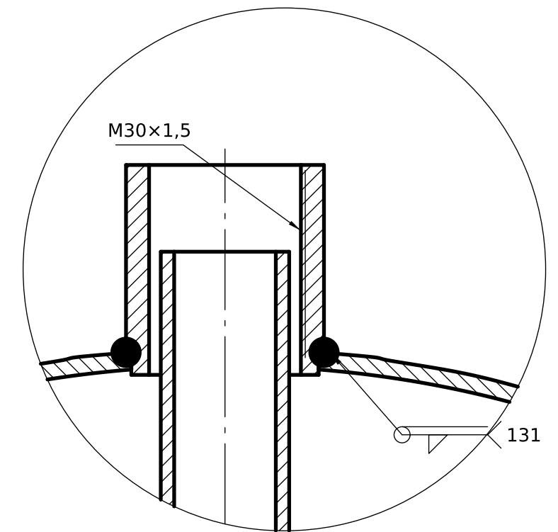
DETALLE B (1:1) Cuello roscado
