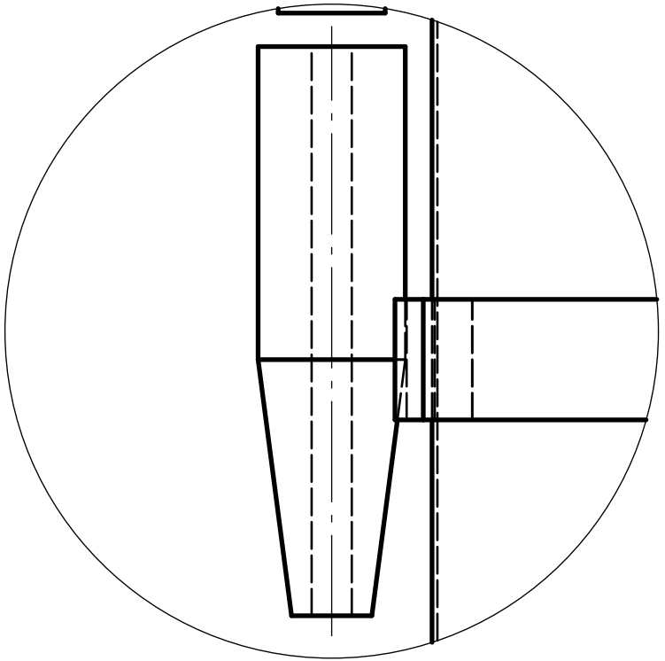
DETALLE E (1:1) Tobera de chorro pleno
