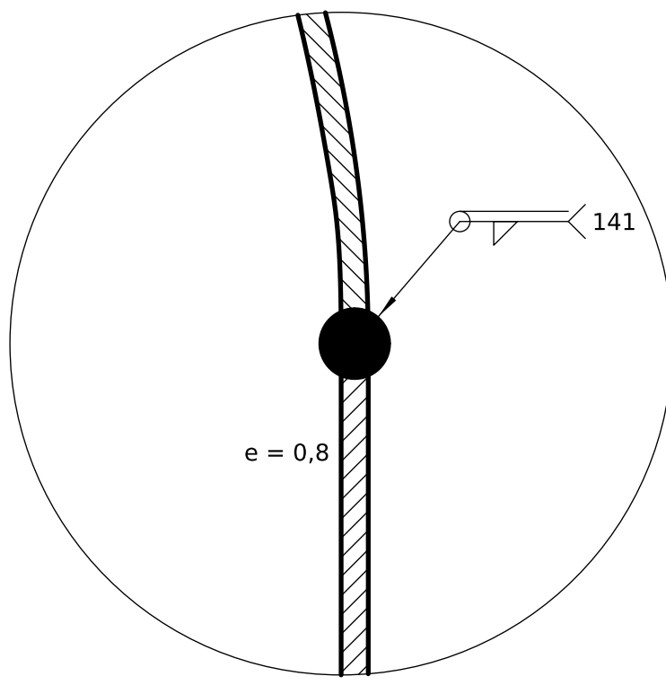
DETALLE C (5:1) Unión cúpula-cuerpo
