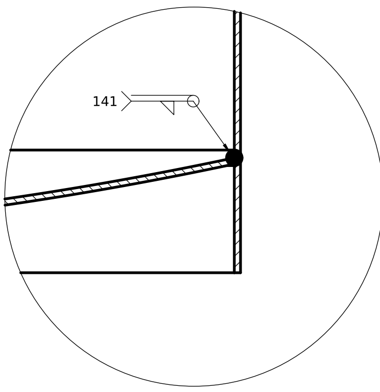
DETALLE D (2:1) Fondo y pollera
