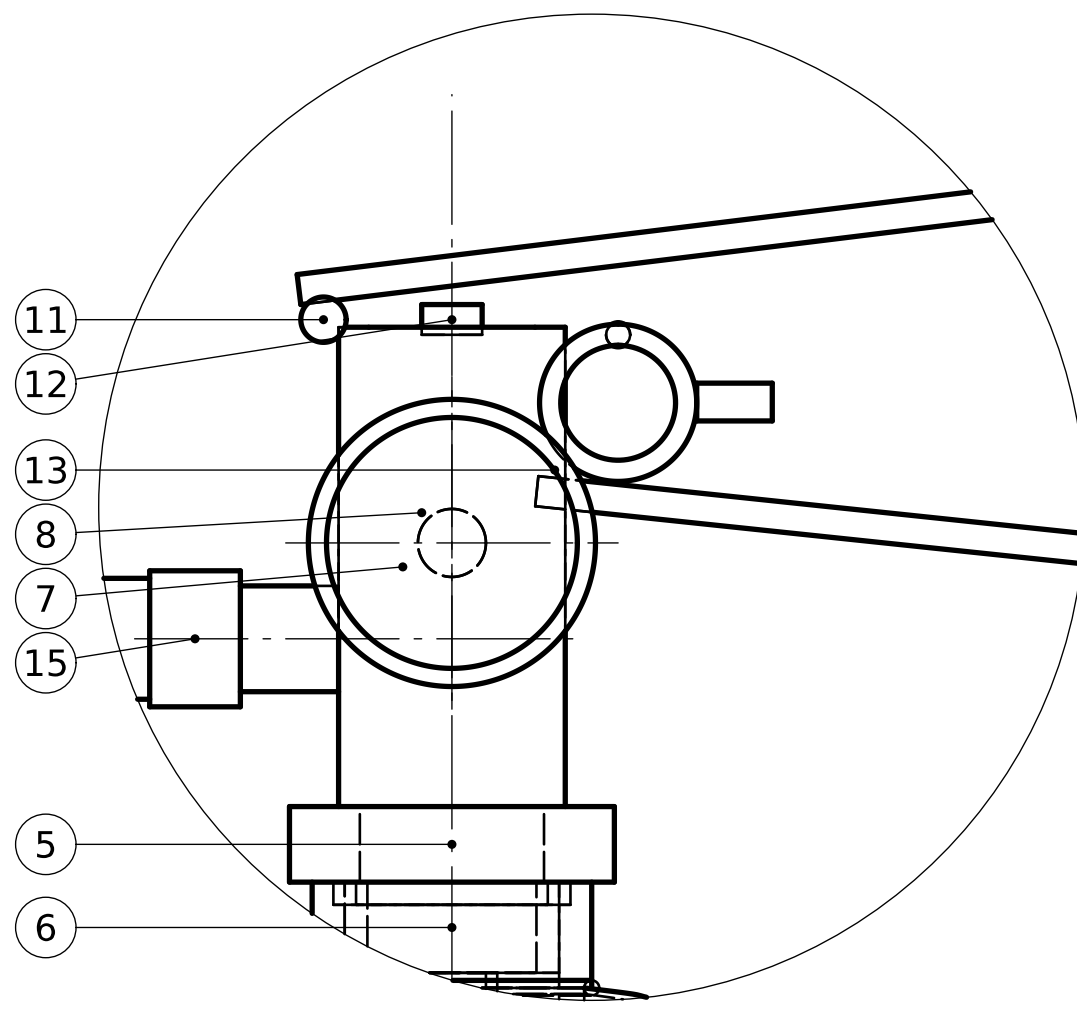
DETALLE A (1:1) Válvula, manómetro y manijas
