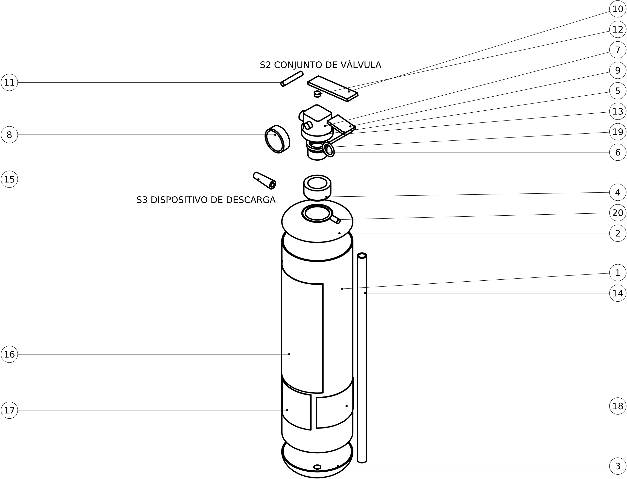
S1 RECIPIENTE (CILINDRO) (FL_REC_ABC_1kg)
