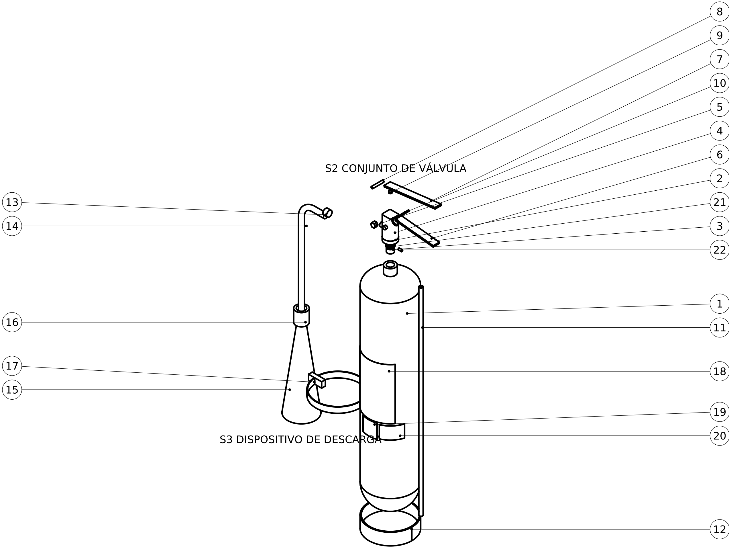
S1 RECIPIENTE (CILINDRO)
