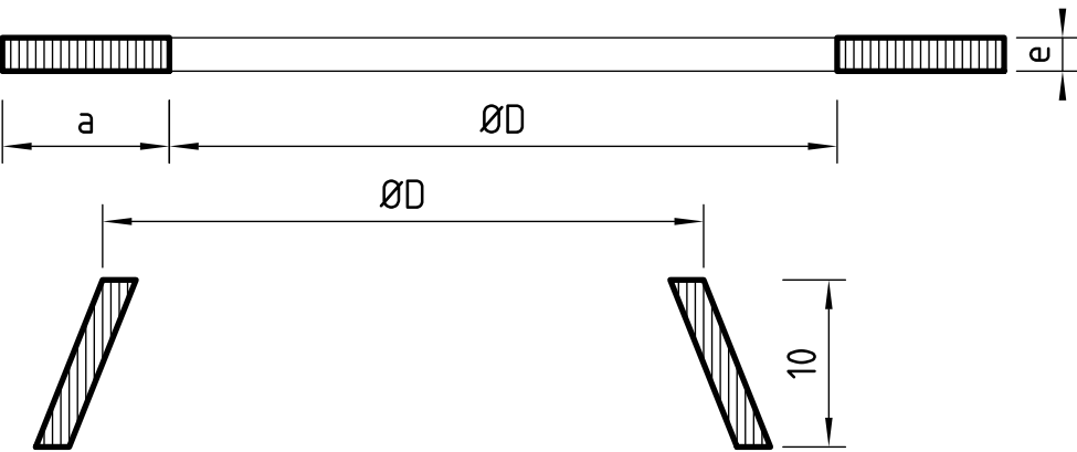
CORTE - anillo cónico
