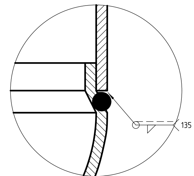
DETALLE D (1:1) Casquete inferior con borde reducido
