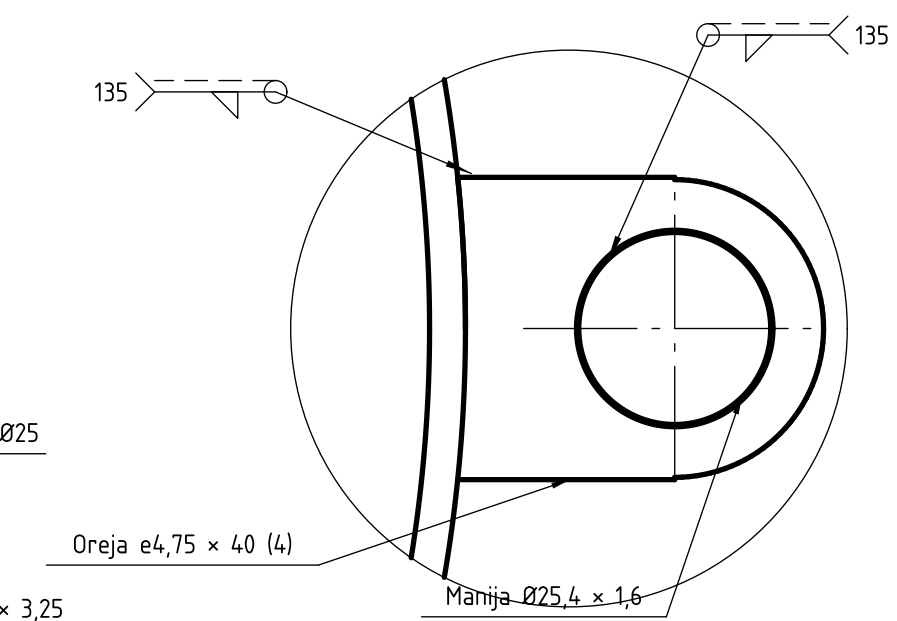
DETALLE G (1:1) Oreja de la manija (vista superior)
