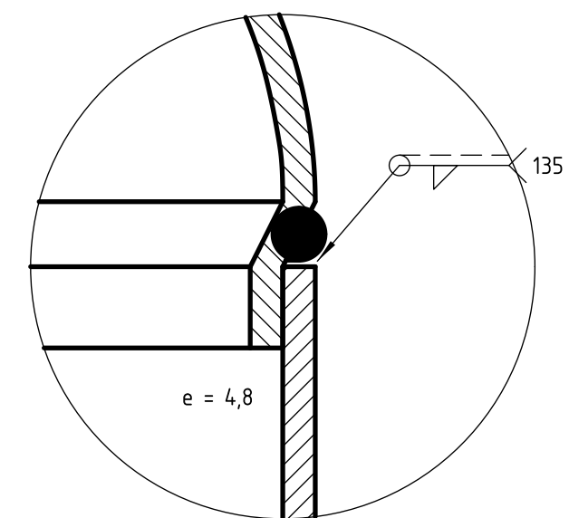
DETALLE C (1:1) Casquete con borde reducido y tope
