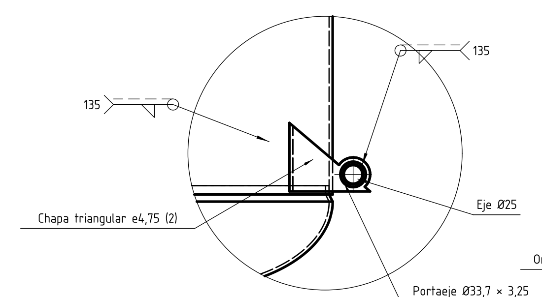
DETALLE F (1:5) Portaeje y chapa triangular (vista lateral, sin rueda)
