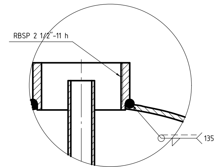
DETALLE B (1:2) Cupla soldada
