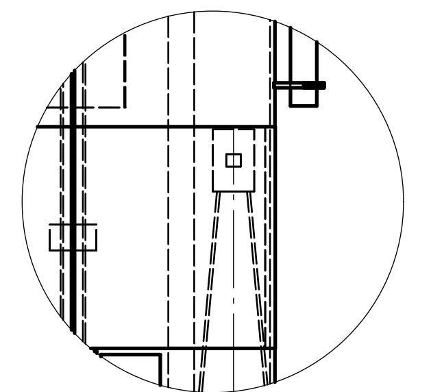
DETALLE E (1:5) Válvula esférica y tobera
