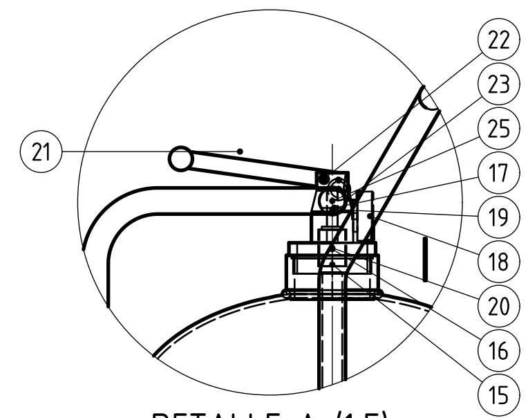
DETALLE A (1:5) Válvula, manómetro y palanca (vista lateral)
