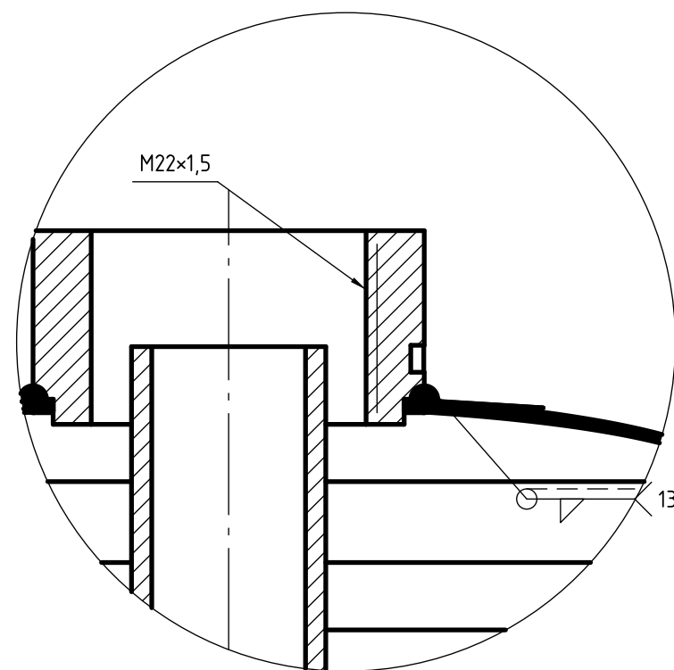
DETALLE B (2:1) Cuello roscado con muesca
