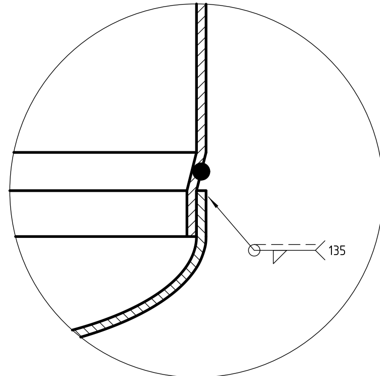
DETALLE D (2:1) Bordón inferior y fondo
