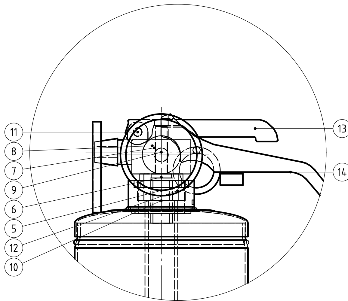
DETALLE A (1:1) Válvula, manómetro y manijas
